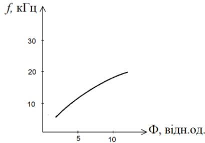
Рис. 2. Вихідна характеристика фотодетектора на одному ОПТ
