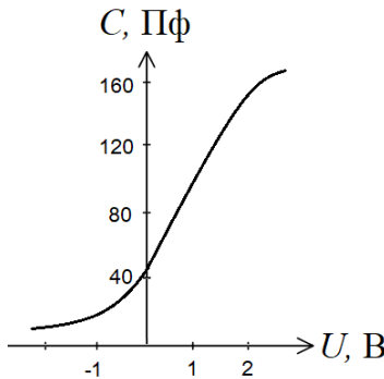
Рис. 5. Залежність ємності МОП-конденсатора від напруги
