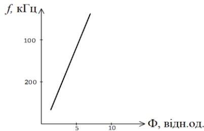
Рис. 6. Залежність вихідної частоти фотодетектора на двох транзисторах та МДП-конденсатором
