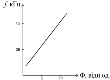
Рис. 4. Вихідна характеристика фотодетектора на двох транзисторах
