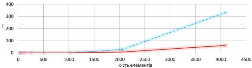
Рисунок 1 – Порівняльний графік результатів множення матриць типу int
