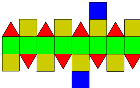
Розгортка псевдоромбокубоктаедра
